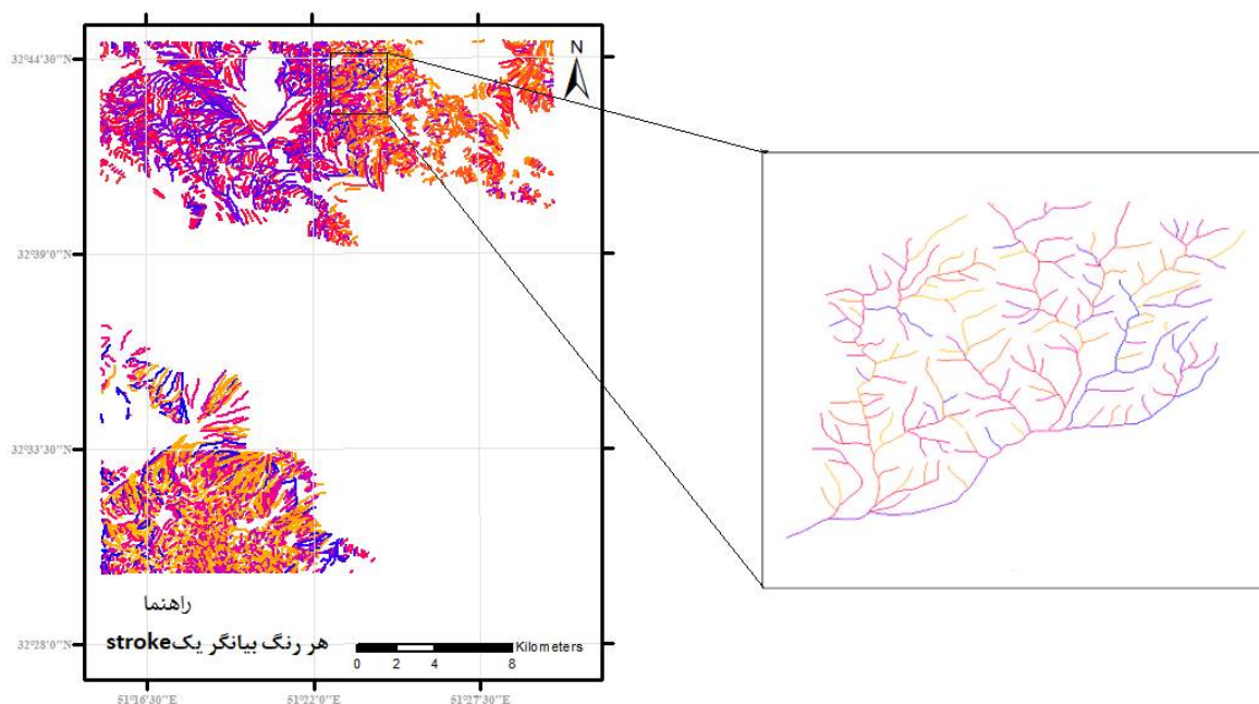
شکل ۱۵- الگوریتم stroke
