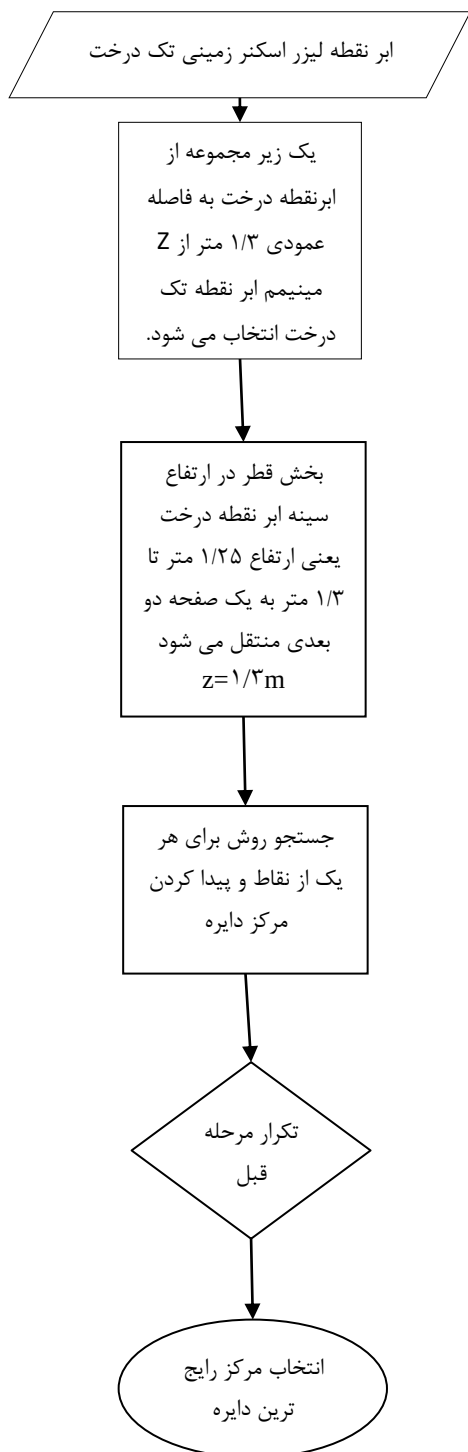
شکل ۷- نمایش فلوچارت الگوریتم انتقال تصادفی هاف
