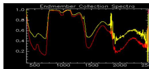
شکل ۵- نمودار حاصل از CR بر روی طیف دارای گرد و غبار و بدون گرد و غبار. منحنی قرمز بدون گرد و غبار و منحنی زرد تحت تأثیر گرد و غبار
