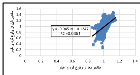
شکل ۷- نمودار تغییرات رفتار باند آبی (BLUE) قبل و بعد از وقوع گرد و غبار
