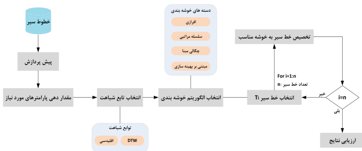
شکل ۲- فلوچارت کلی مقایسه دسته های مختلف خوشه بندی خطوط سیر
