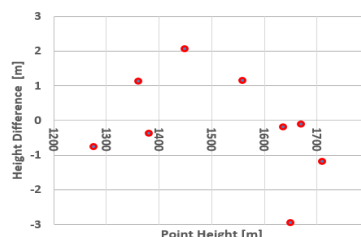
شکل ۵- خطای ارتفاعی SRTM در موقعیت نقاط کنترل زمینی
