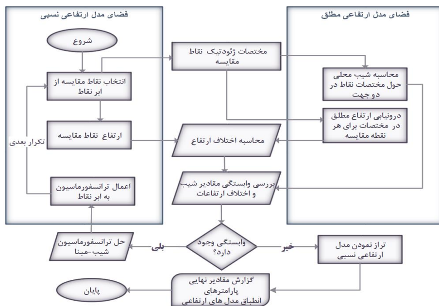
شکل ۱- فلوچارت روش پیشنهادی انطباق مدل‌های ارتفاعی
