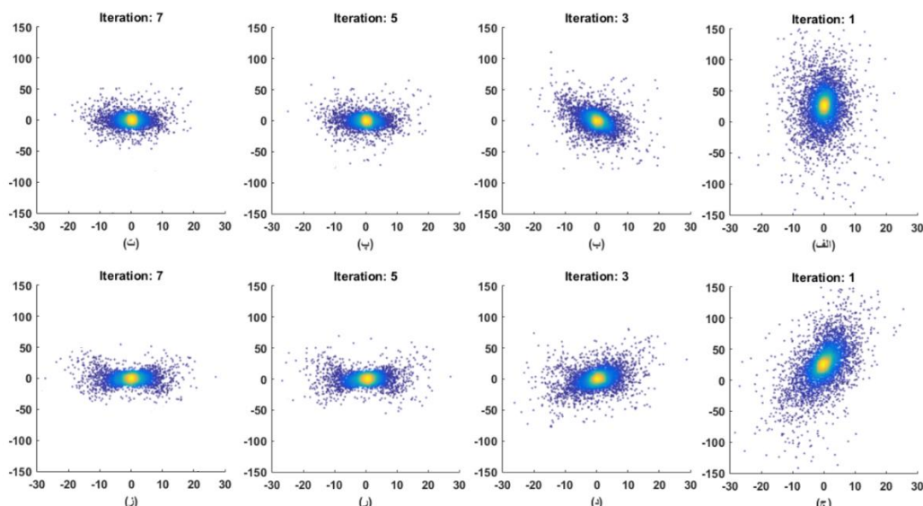
شکل ۷- تکرارهای مرحله ترانسفورماسیون شیب-مبنا در تناظریابی دو مدل نسبی MATDEM و مدل مطلق SRTM. کاهش تدریجی وابستگی اختلاف ارتفاع دو مدل: (الف) تا (ت) نسبت به شیب محلی در امتداد طول ژئودتیک، (ج) تا (ز) نسبت به شیب محلی در امتداد عرض ژئودتیک
