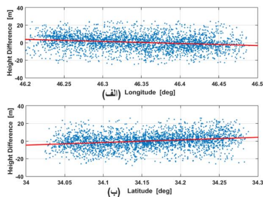
شکل ۸- (الف) وابستگی اختلاف ارتفاع باقیمانده به طول ژئودتیک نقاط پس از حل پارامترهای ترانسفورماسیون شیب-مبنا (ب) وابستگی اختلاف ارتفاع باقیمانده به عرض ژئودتیک نقاط پس از حل وابستگی به طول ژئودتیک
