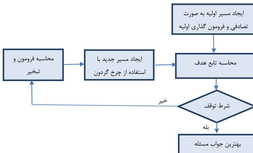
شکل ۴- نمودار چرخه کار الگوریتم مورچگان
