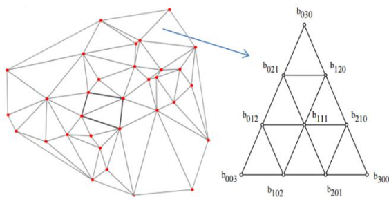
شکل ۲- نمایش المان مثلثی بزرگ کوبیک
