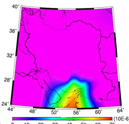
شکل ۸- نمایش تغییرات ماکزیمم برش در نقاط مختلف شبکه
