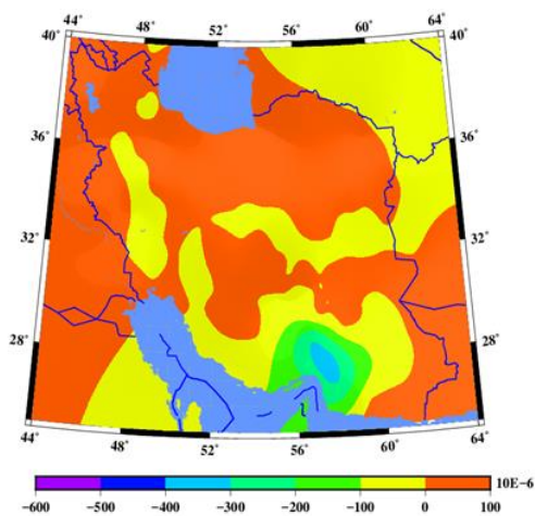
شکل ۷- نمایش تغییرات کمیت اتساع در نقاط مختلف شبکه
