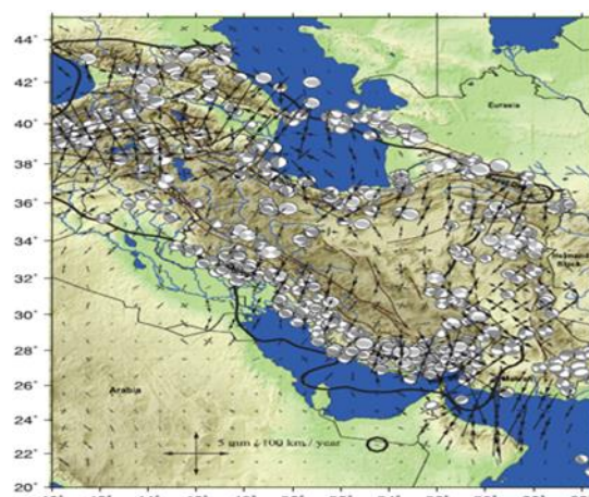
شکل ۱۰- تانسور نرخ استرین و مکانیزم لرزه‌ای [۹]
