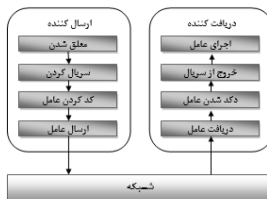
شکل ۴- مراحل انتقال عامل در شبکه [۹]
