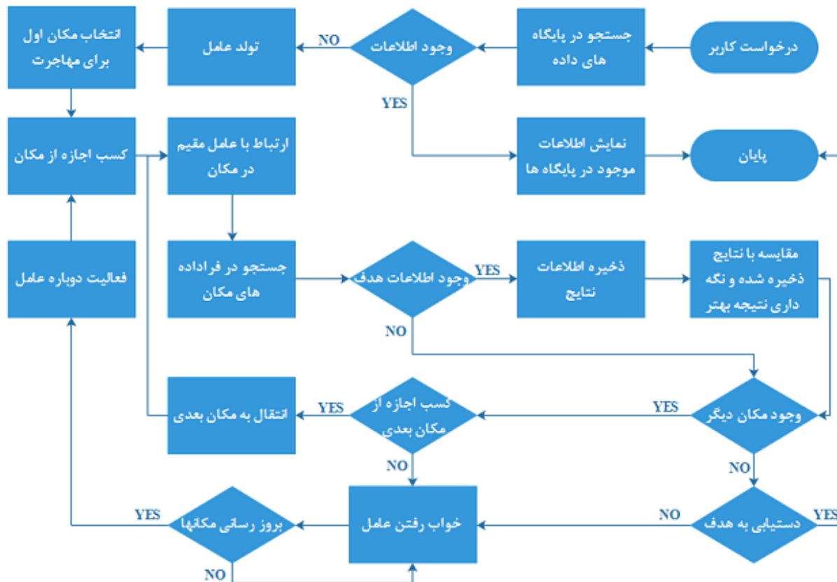
شكل ٧- الگوریتم سیستم عامل سیار
