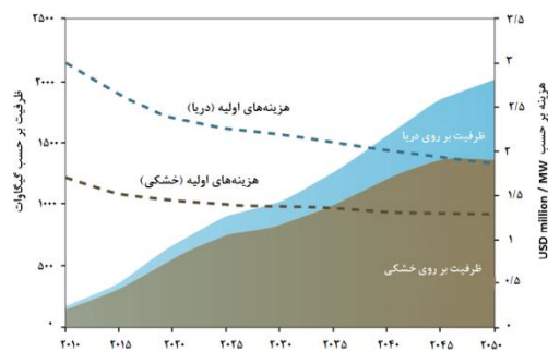
شکل ۴- ظرفیت توسعه انرژی بادی و کاهش قیمت‌های مربوط به آن در سال‌های ۲۰۵۰ تا ۲۰۰۸ [۳]
