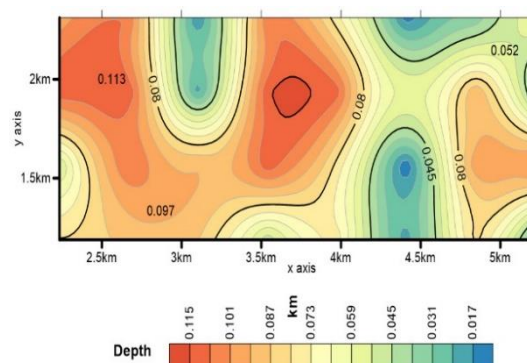
شکل ۷- نقشه منحنی میزان عمق منشورها تولید شده در حالت بدون نویز
