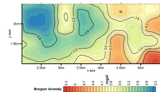
شکل ۵- نقشه آنومالی بوگه در حالت بدون نویز
