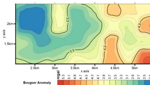
شکل ۶- نقشه آنومالی بوگه در حالت دارای نویز
