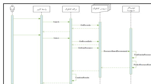
شکل ۵- نمودار توالی روال توصیه‌گری منبع‌منا در درگاه مکانی توصیه‌گر
