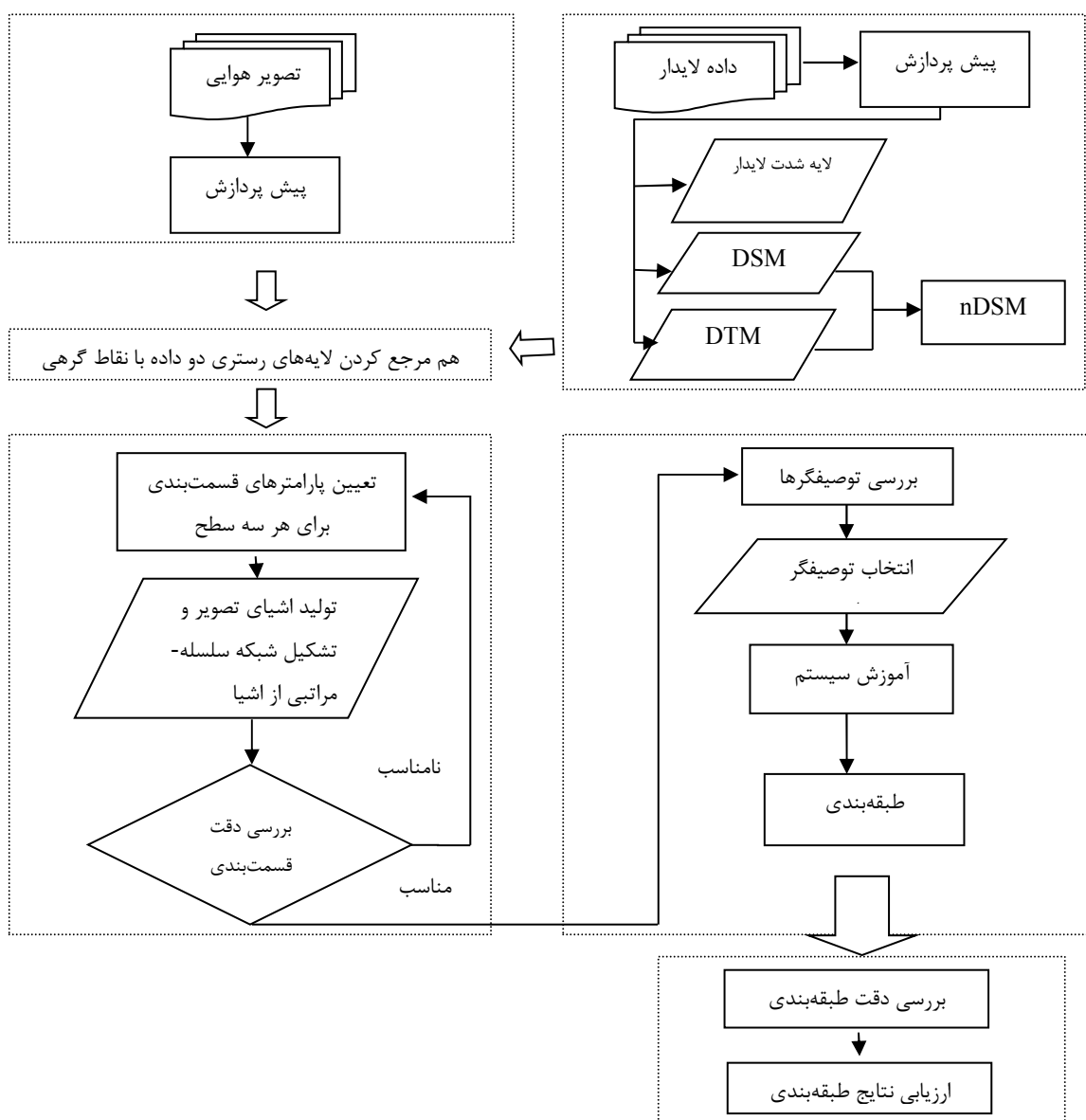
شکل ۳- فلوچارت کلی روش پیشنهادی
