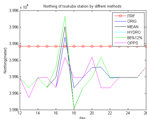
شکل ۳- مؤلفه‌ی شمالی محاسبه شده با پنج روش متفاوت
