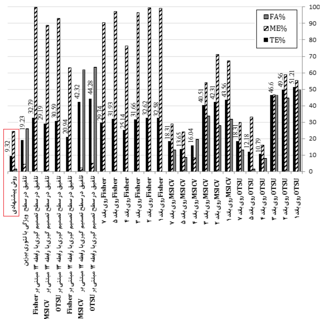
شکل ۶- پارامترهای کمی صحت آشکارسازی تغییرات به روش‌های: حدآستانه گذاری تک بعدی OTSU، MSICV و Fisher بر روی باندهای اصلی تصویر اختلاف قدرمطلق، به همراه نتایج حاصل از حدآستانه گذاری چندبندی مبتنی بر تلفیق داده‌ها در سطح تصمیم گیری با روابط (۱۲) و (۱۳)، تلفیق در سطح ویژگی با تئوری بیزین و نتایج حاصل از روش پیشنهادی.
