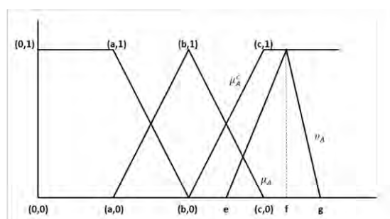
شکل ۱- عدد فازی شهودی مثلثی A = (\langle a, b, c \rangle, \langle e, f, g \rangle)
