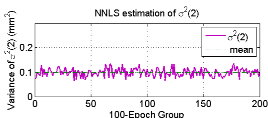
شکل ۲- برآورد کمترین مربعات مولفه‌های وریانس
