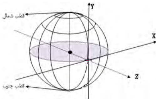
شکل ۲- نمایش سیستم مختصات ژئودتیک محلی
